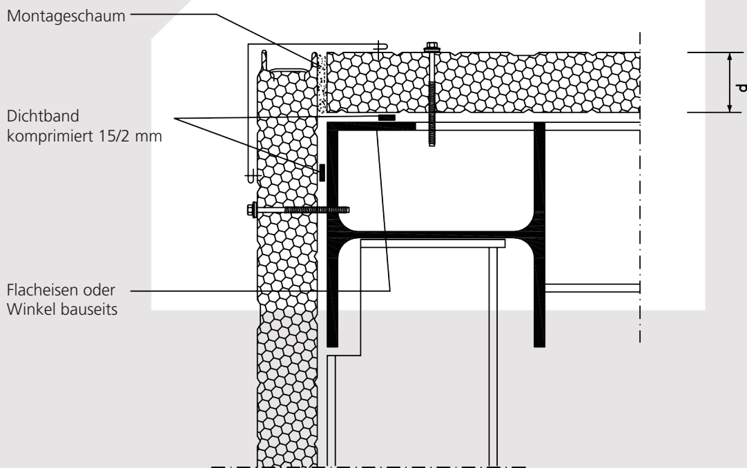
HORIZONTALSCHNITTE
