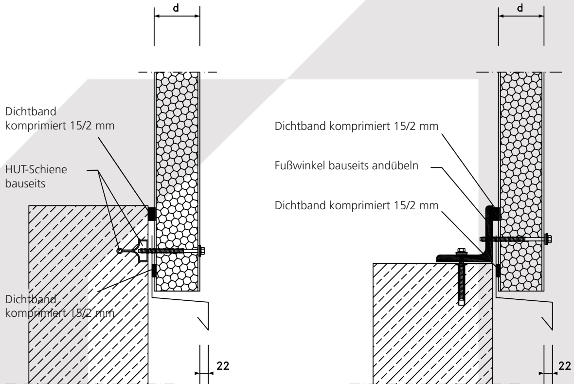
VERTIKALSCHNITT
